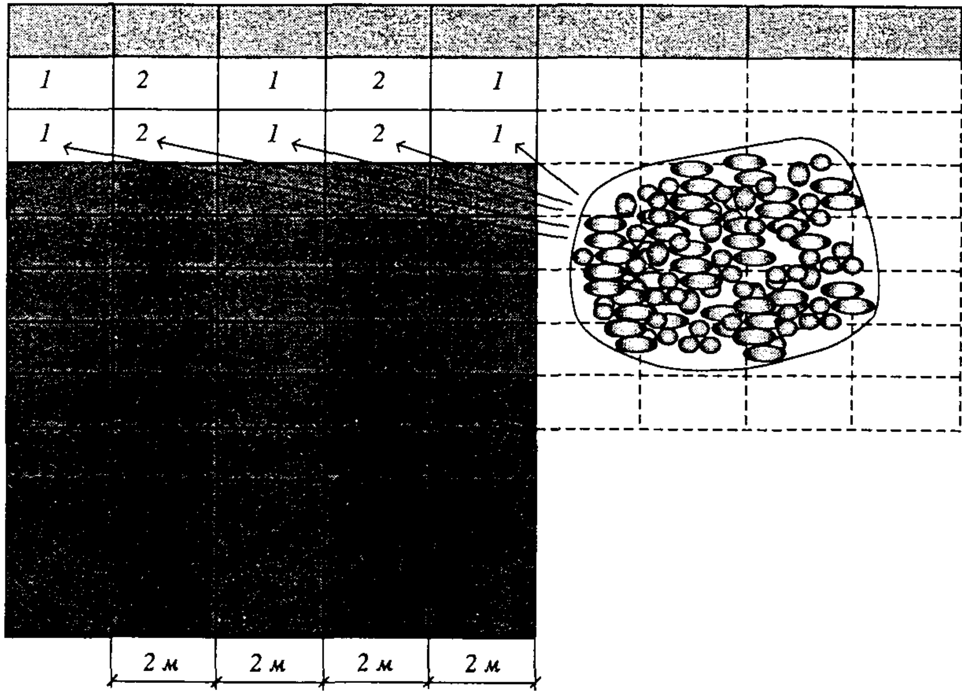
Рис. 4.7. Схема заполнения стыковых секций камнем: 1, 2 – очередность заполнения
