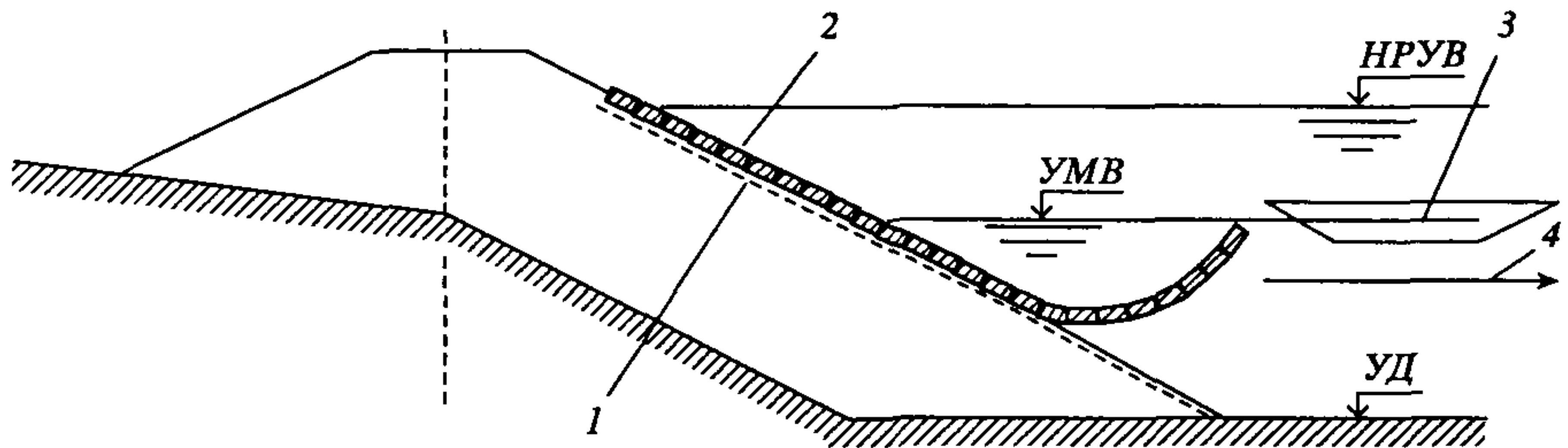
Рис. 4.7. Схема заполнения стыковых секций камнем: 1, 2 – очередность заполнения
