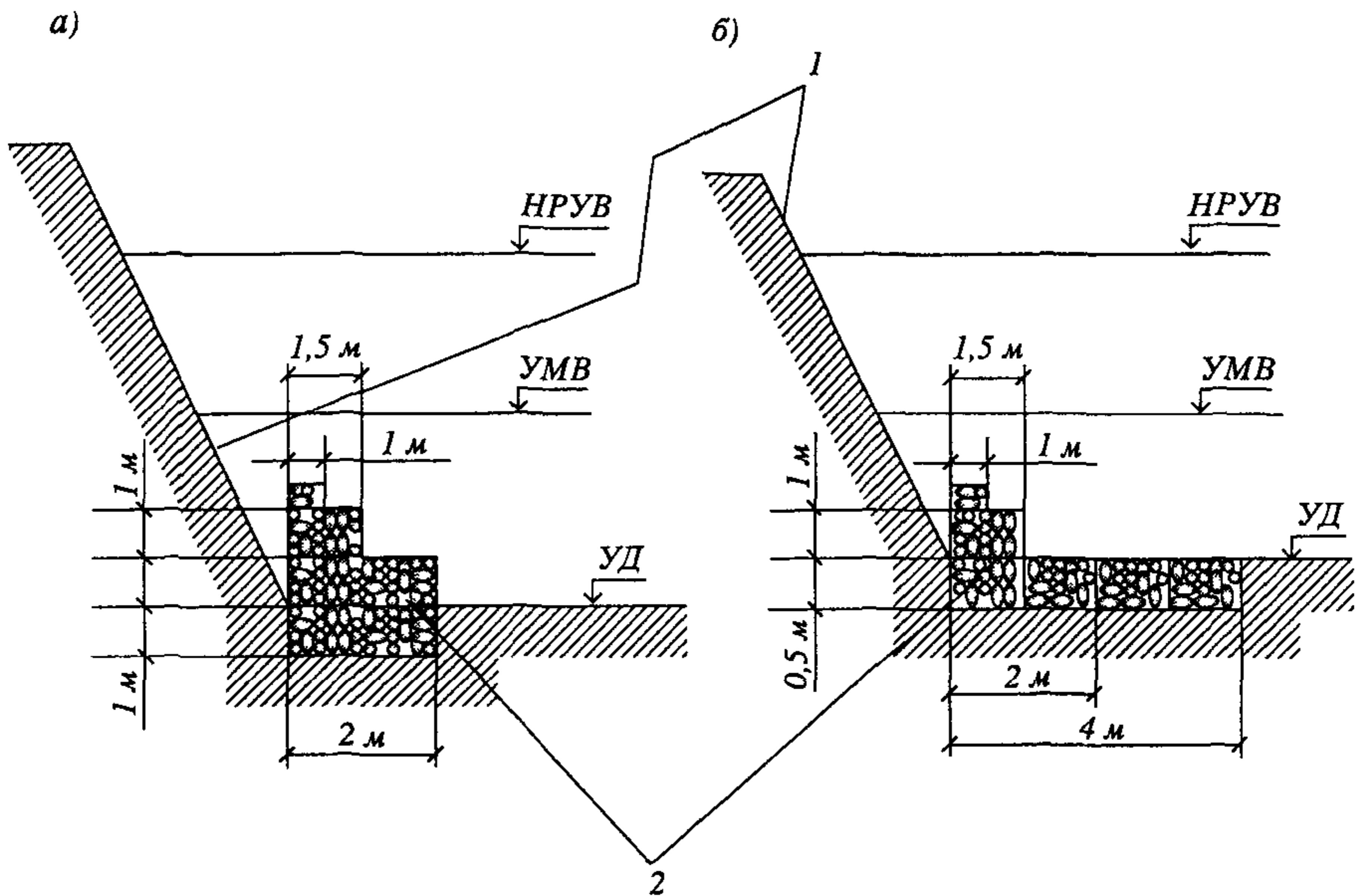
Рис. 4.18. Схема установки блоков габиона стены:
