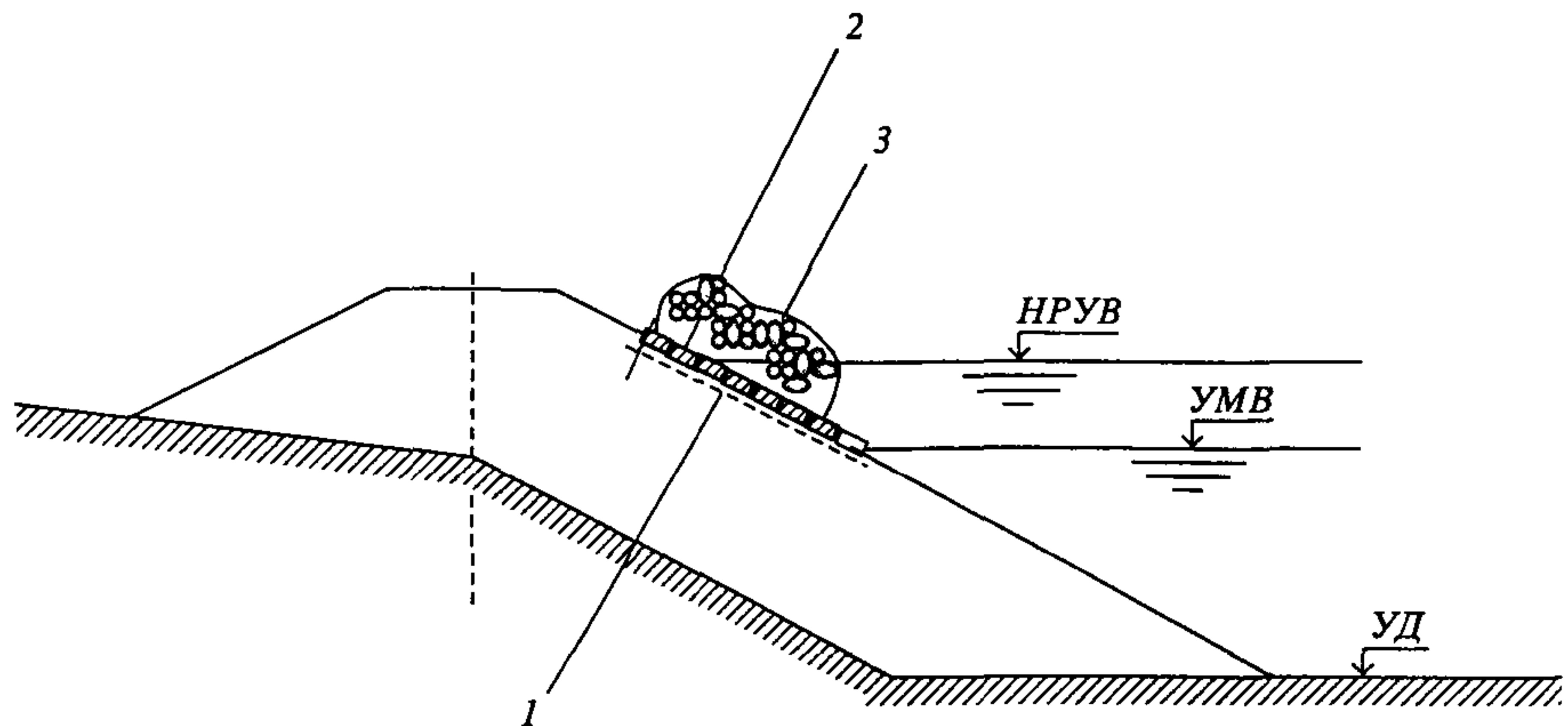
Рис. 4.1. Схема выгрузки камня (первая стадия строительства):
