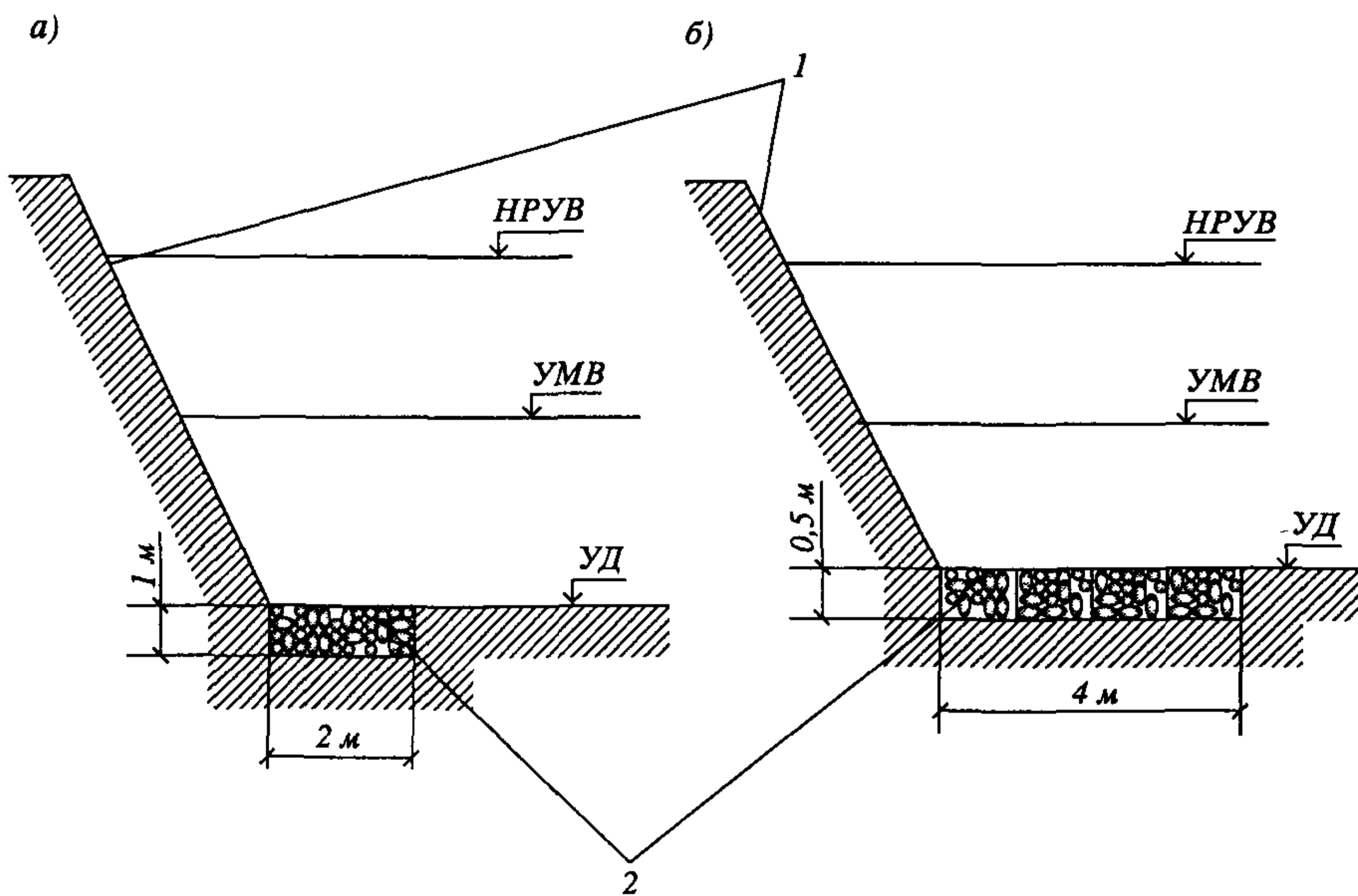
Рис. 4.17. Схема установки фундаментальных блоков габионов:
