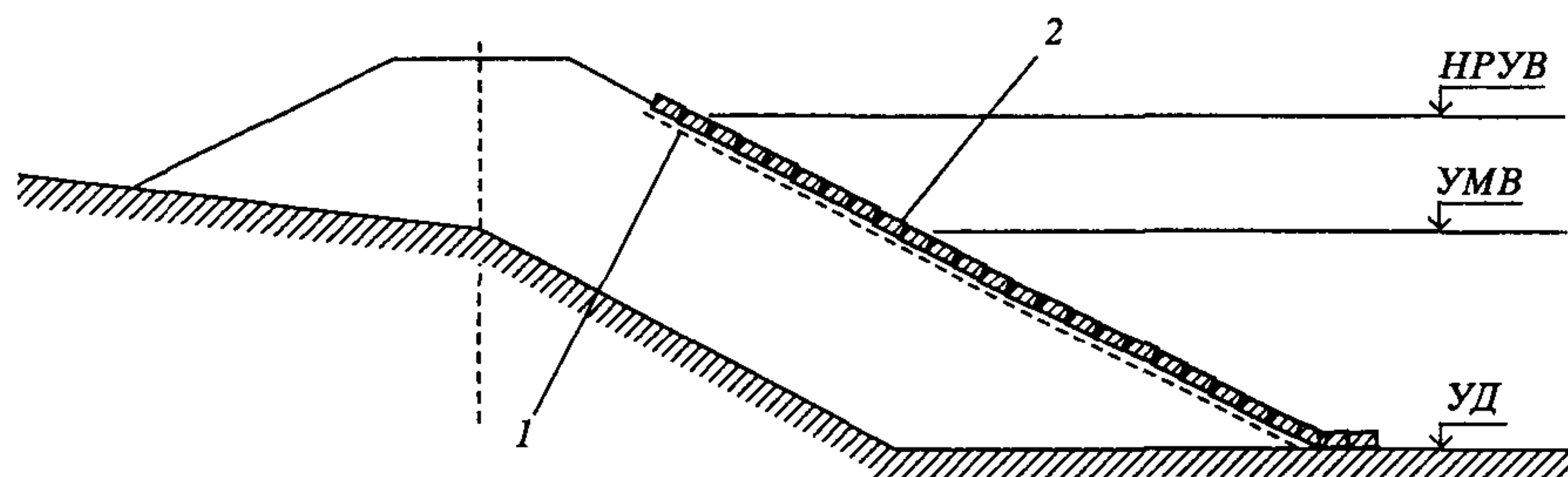
Рис. 4.11. Проектное положение габионной структуры на откосе:
