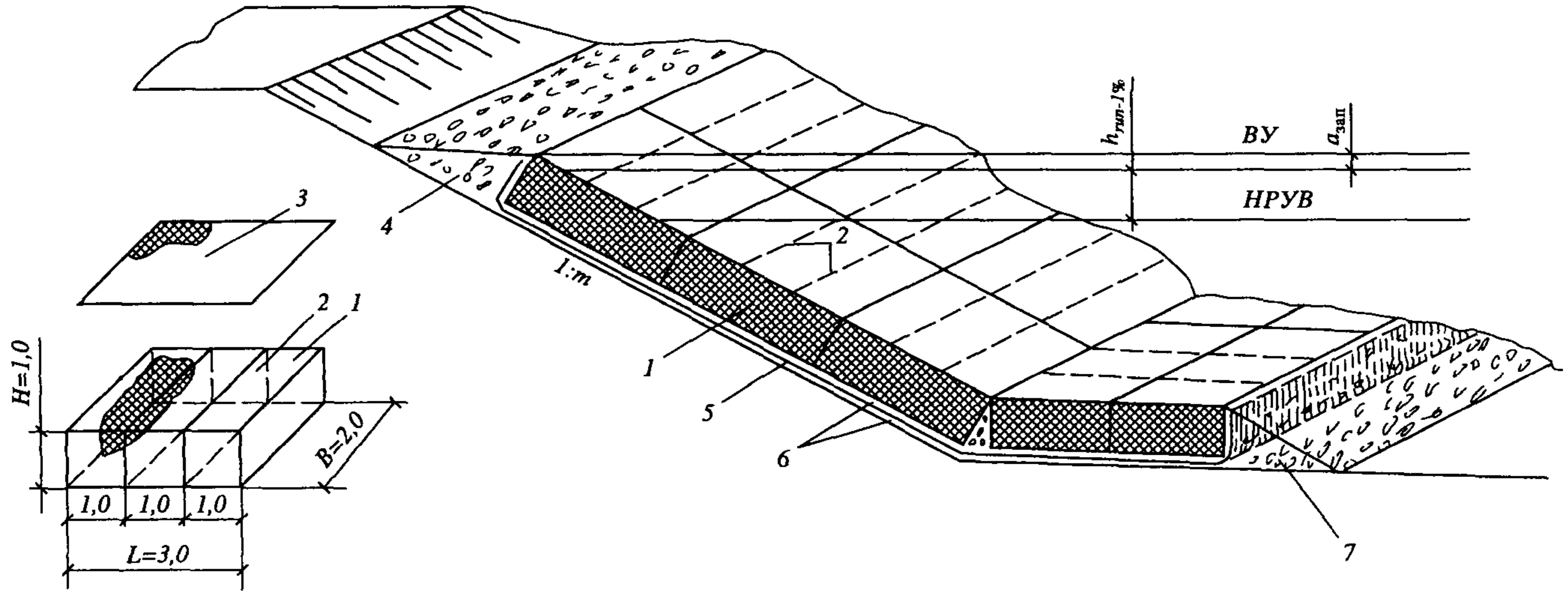
Лист. 5. Однослойная защита из габионов с диафрагмами МД2, H = 1,0 м
