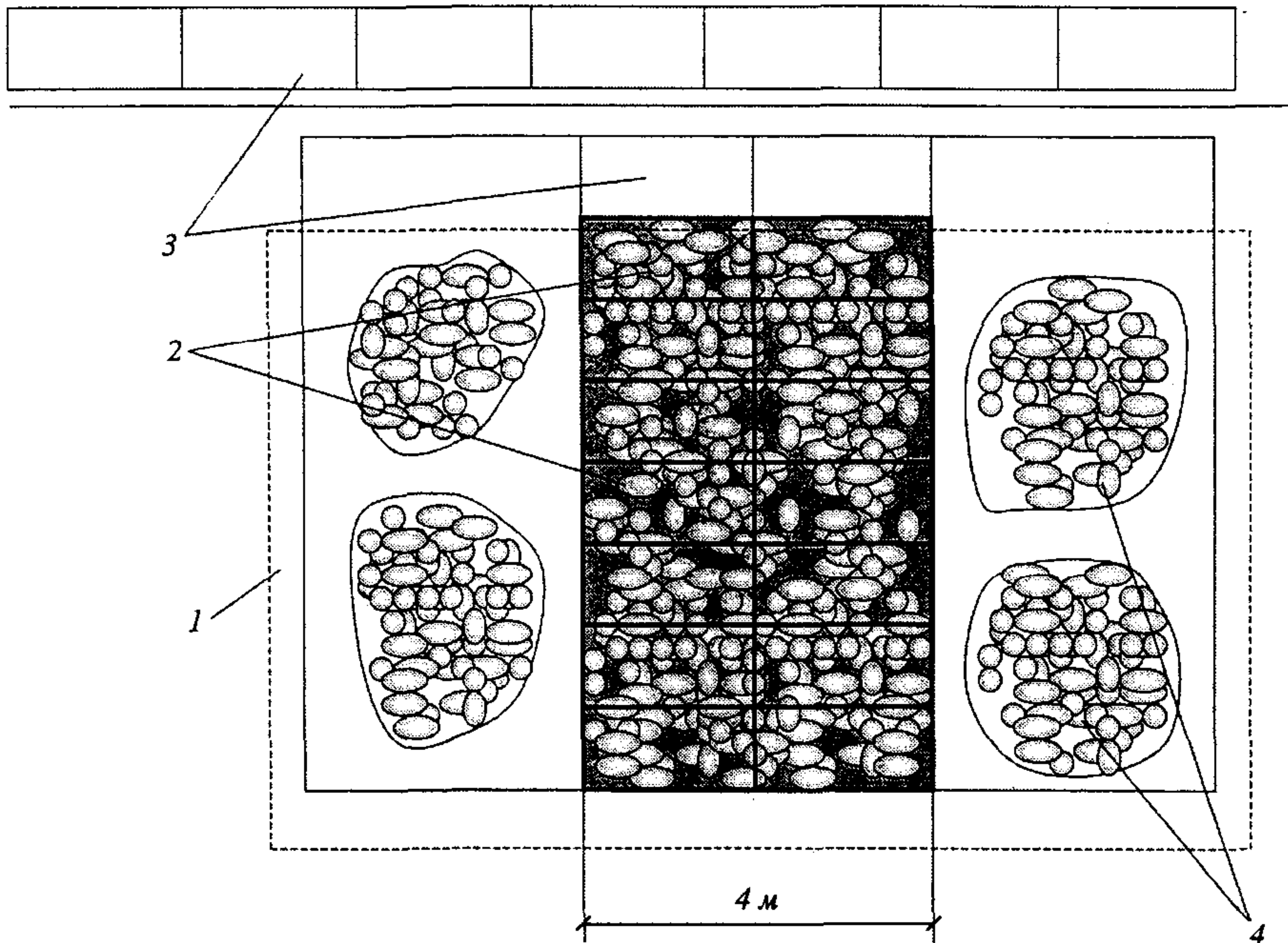
Рис. 4.4. Схема размещения конструкций на понтоне:
