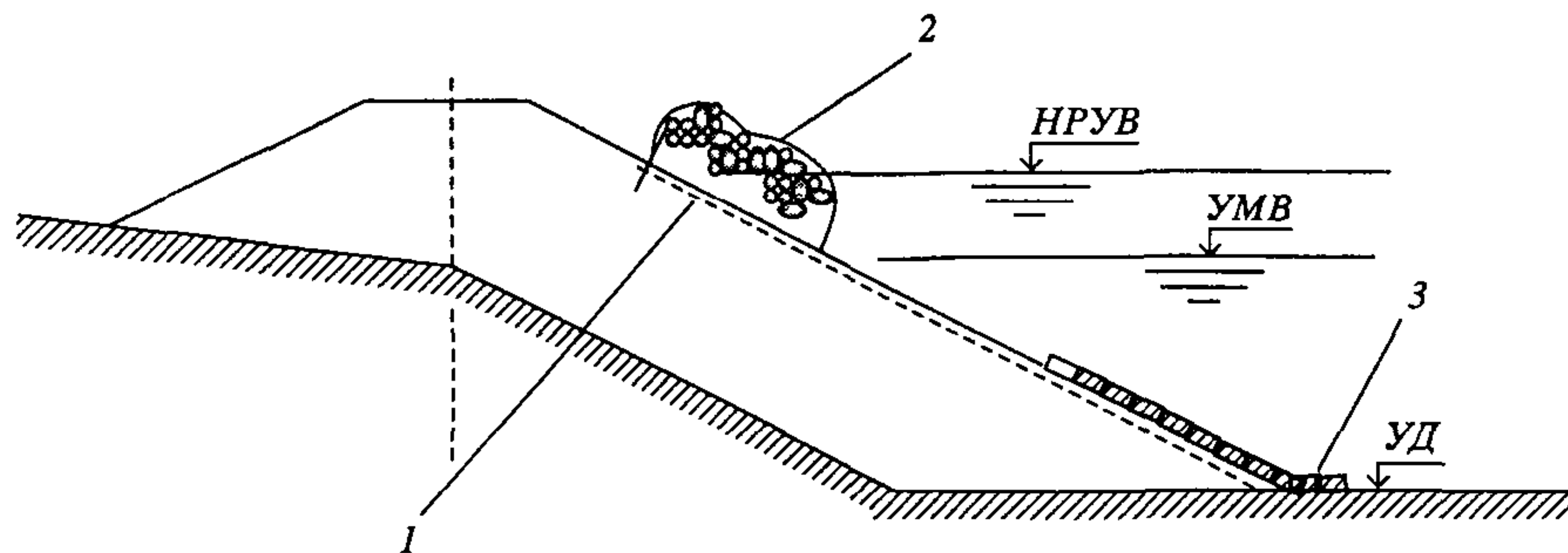
Рис. 4.10. Схема выгрузки камня на откосе:
