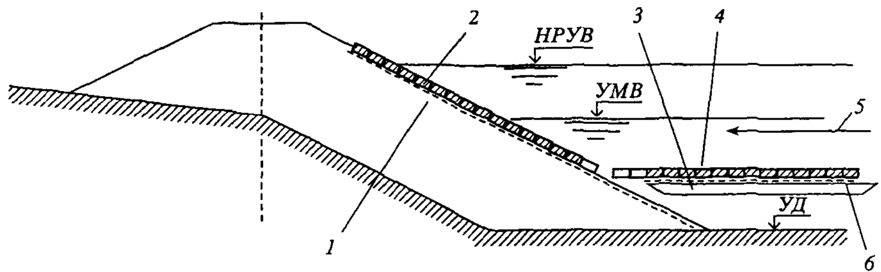
Рис. 4.5. Схема подвода системы габионов к откосу на понтоне:
