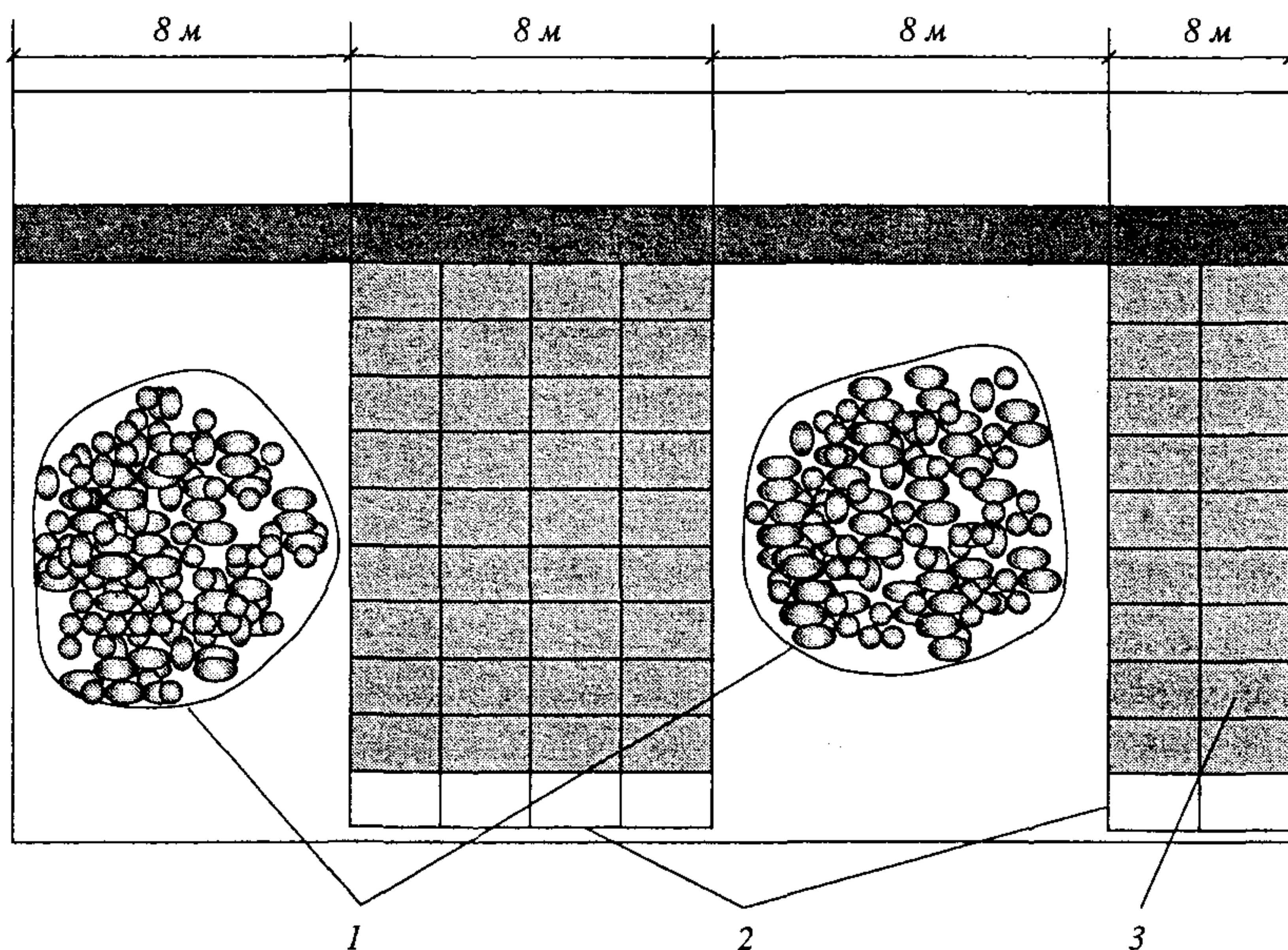
Рис. 4.2. План-схема выгрузки камня:
