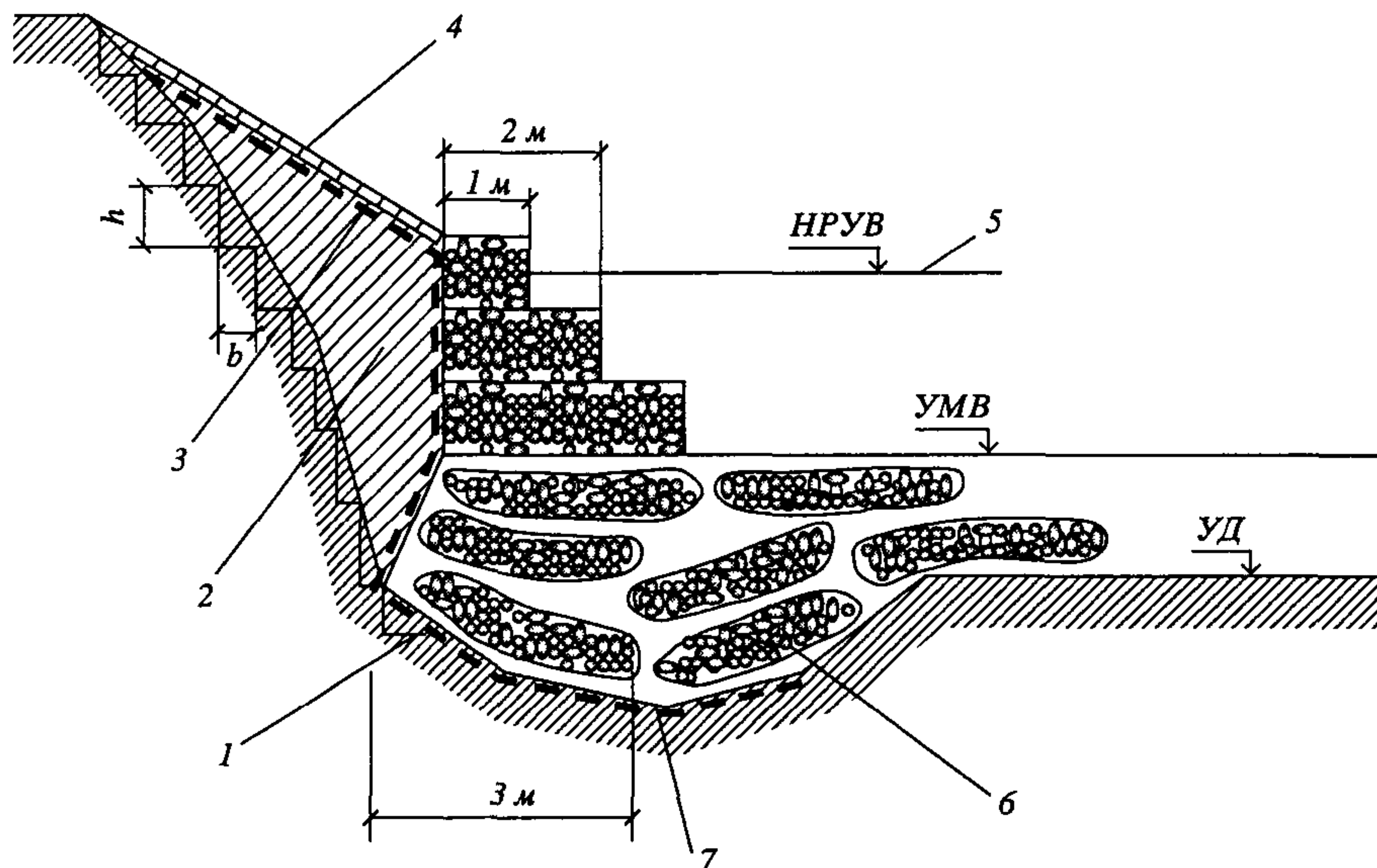
Рис. 4.15. Проектное положение конструкции:
