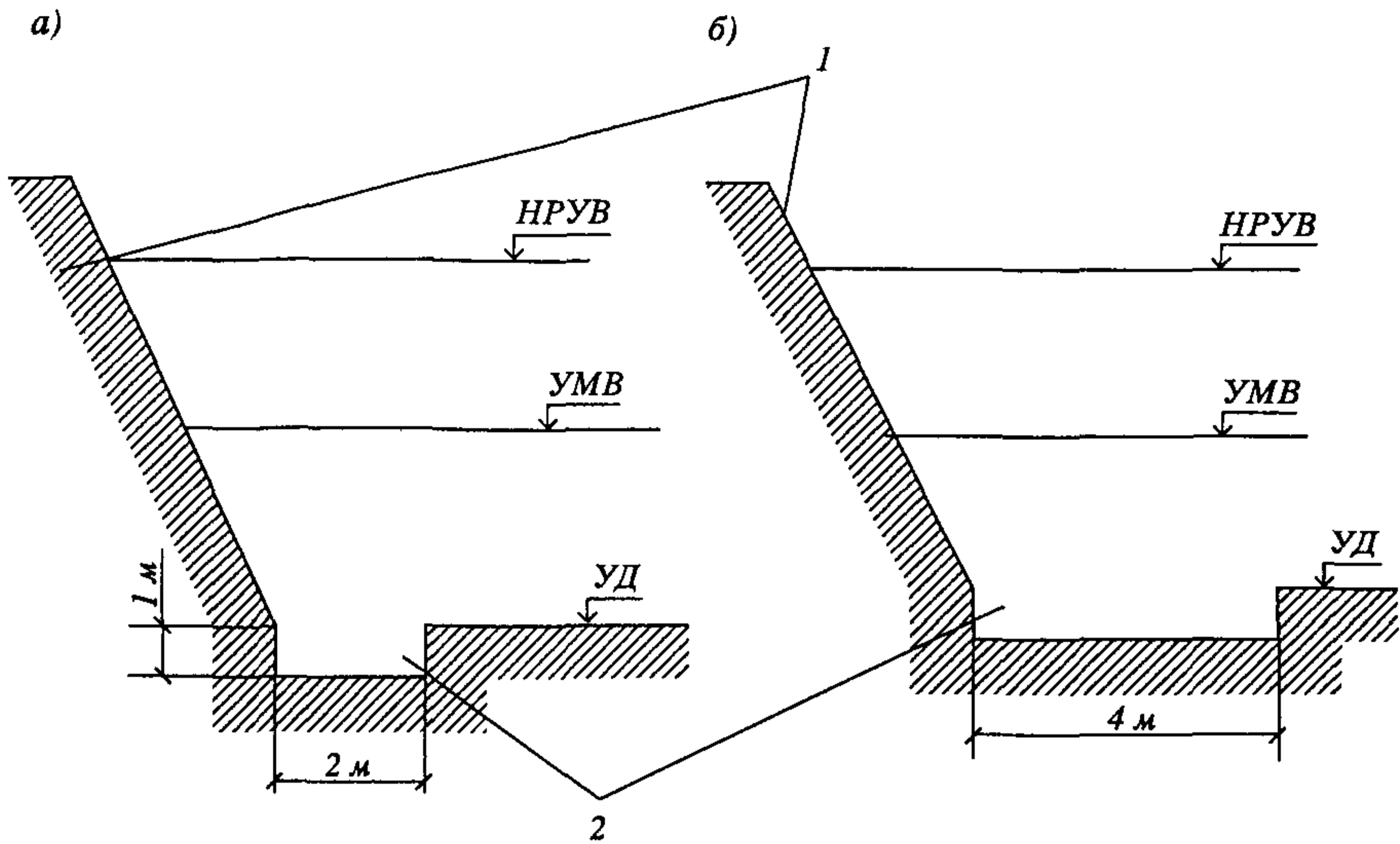
Рис. 4.16. Схема устройства траншеи вдоль откоса:
